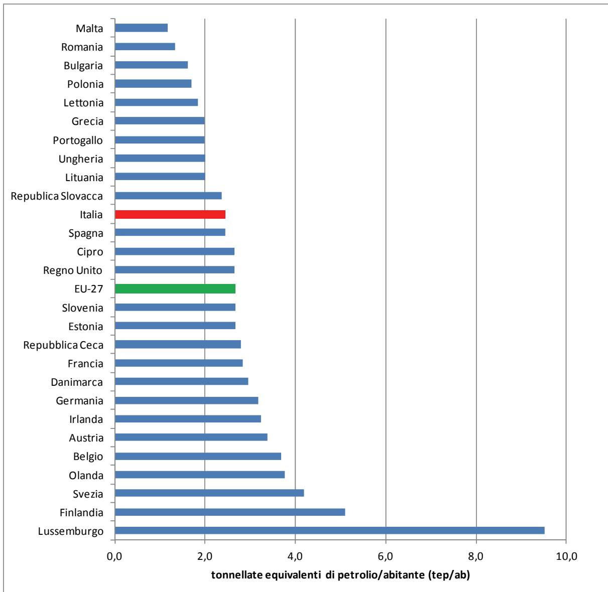
Figura 20: Consumo finale di energia per abitante – Anno 2009
