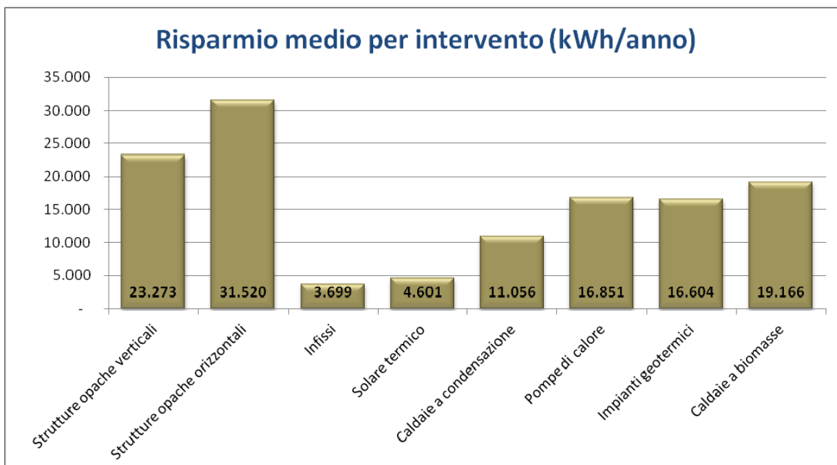
FIG. 8: RISPARMIO MEDIO ANNUO ASSOCIATO ALLA SINGOLA TIPOLOGIA DI INTERVENTO. VALORI ESPRESSI IN KWh/ANNO – REGIONE PIEMONTE , ANNO 2010
