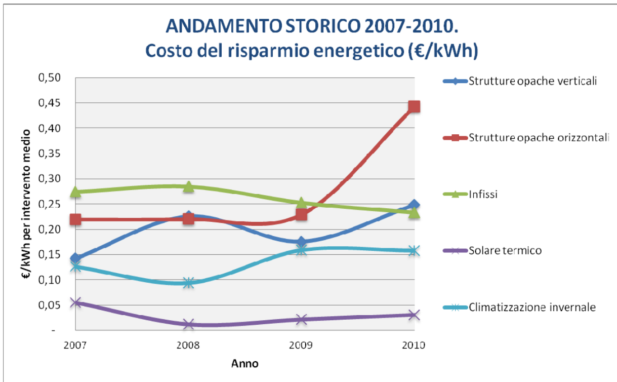
FIG. 11: REGIONE CALABRIA DATI STORICI ANNI 2007-2010: ANDAMENTO DEL COSTO DEL RISPARMIO ENERGETICO UNITARIO DISTINTO PER TIPOLOGIA DI INTERVENTO. VALORI ESPRESSI IN €/kWh
