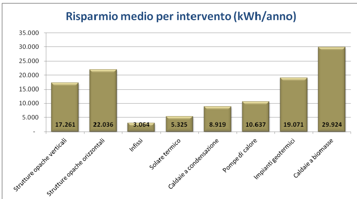
FIG. 8: RISPARMIO MEDIO ANNUO ASSOCIATO ALLA SINGOLA TIPOLOGIA DI INTERVENTO. VALORI ESPRESI IN KWh/ANNO – REGIONE EMILIA-ROMAGNA, ANNO 2010
