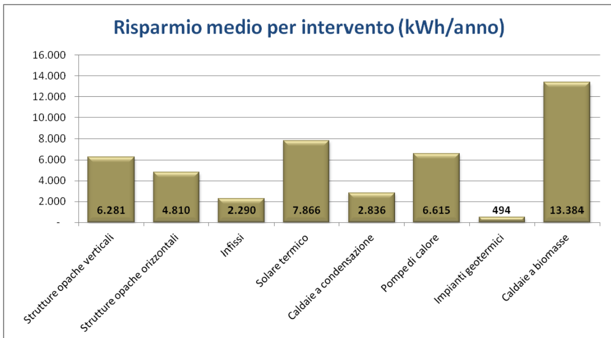
FIG. 8: RISPARMIO MEDIO ANNUO ASSOCIATO ALLA SINGOLA TIPOLOGIA DI INTERVENTO. VALORI ESPRESSI IN KWh/ANNO – REGIONE CALABRIA, ANNO 2010
