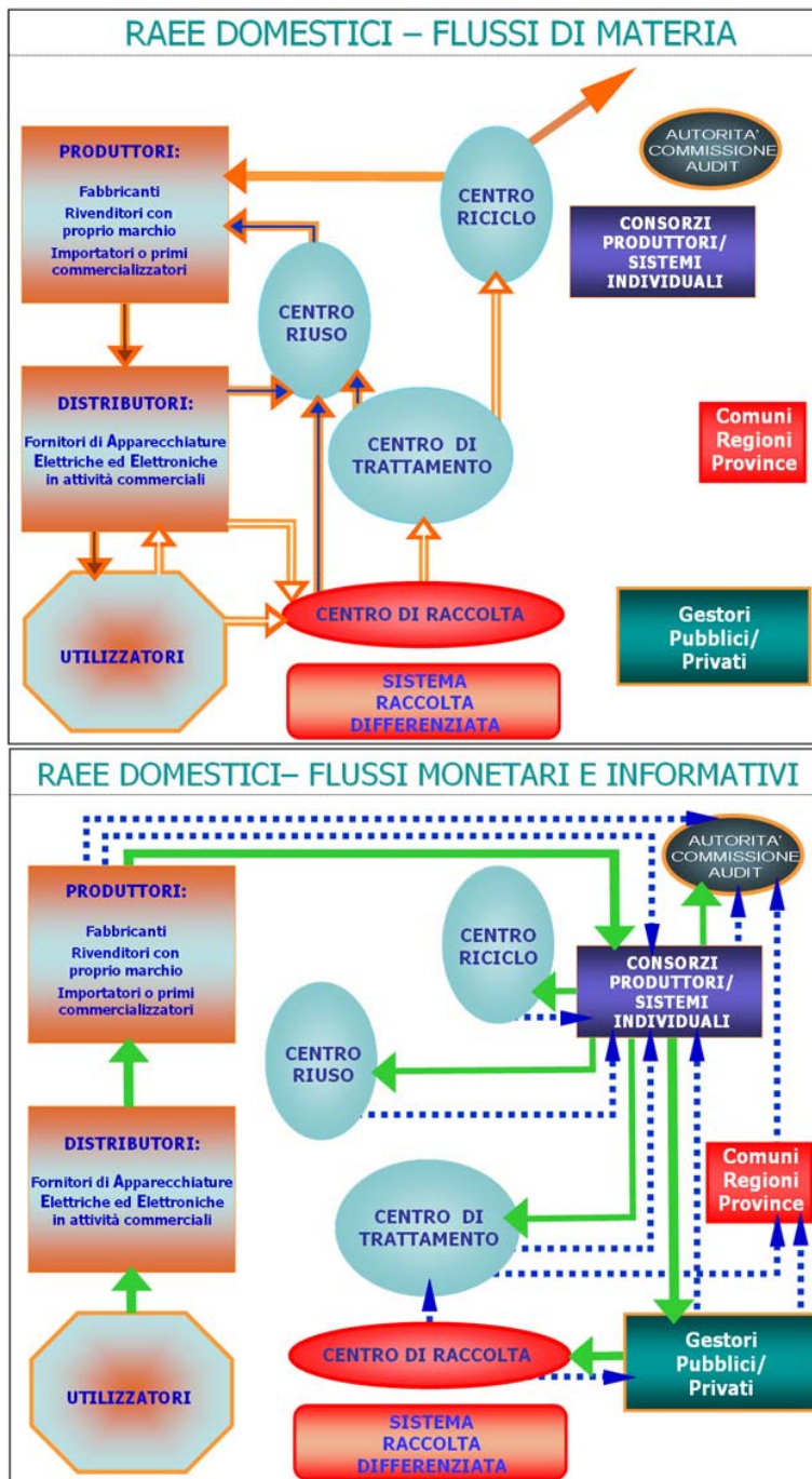
Fig.4 – Schemi di principio dei sistemi di raccolta apparecchiature elettriche ed elettroniche. In alto i flussi di materia, le frecce a riempimento marrone si riferiscono alle apparecchiature da immettere alla vendita, quelle a riempimento bianco alle apparecchiature usate, quelle a riempimento blu alle apparecchiature di cui è possibile il reimpiego, quelle uniformi ai residui da avviare a smaltimento. In basso i flussi monetari (linee verdi) ed i flussi informativi (linee a tratteggio blu).
