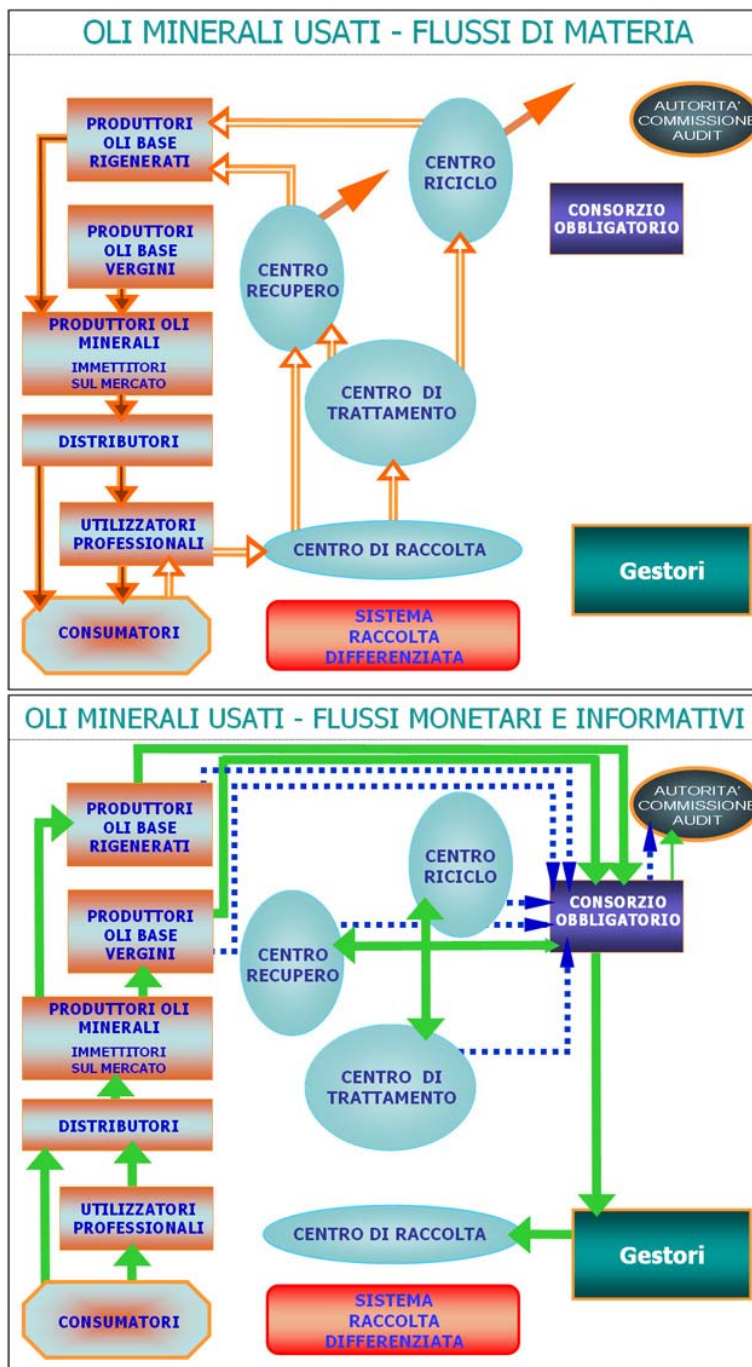
Fig. 3 – Schemi di principio del sistema consortile per la gestione, raccolta e trattamento degli oli minerali usati. In alto i flussi di materia, le frecce a riempimento marrone si riferiscono agli oli da immettere alla vendita, quelle a riempimento bianco agli oli usati, quelle uniformi ai residui da avviare a smaltimento. In basso i flussi monetari riferiti al Consorzio obbligatorio (linee verdi) ed i flussi informativi (linee a tratteggio blu).
