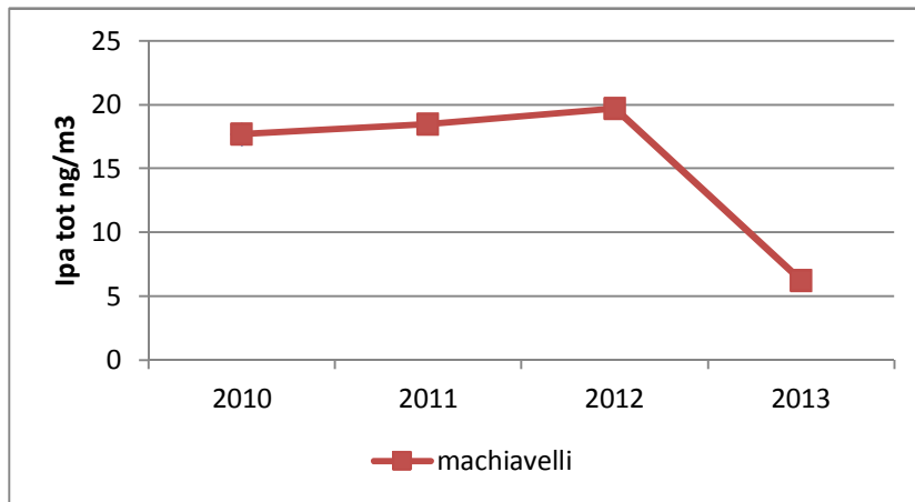
Fig.12 - Medie annuali IPAtot nella stazione di Machiavelli
