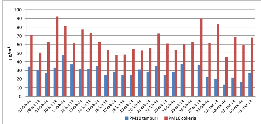
Fig.18 – Misure di PM10 Tamburi vs Cokeria
