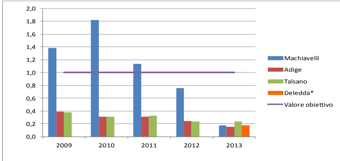
Fig.7 - Medie annuali BaP (ng/m3) in tutti i siti
