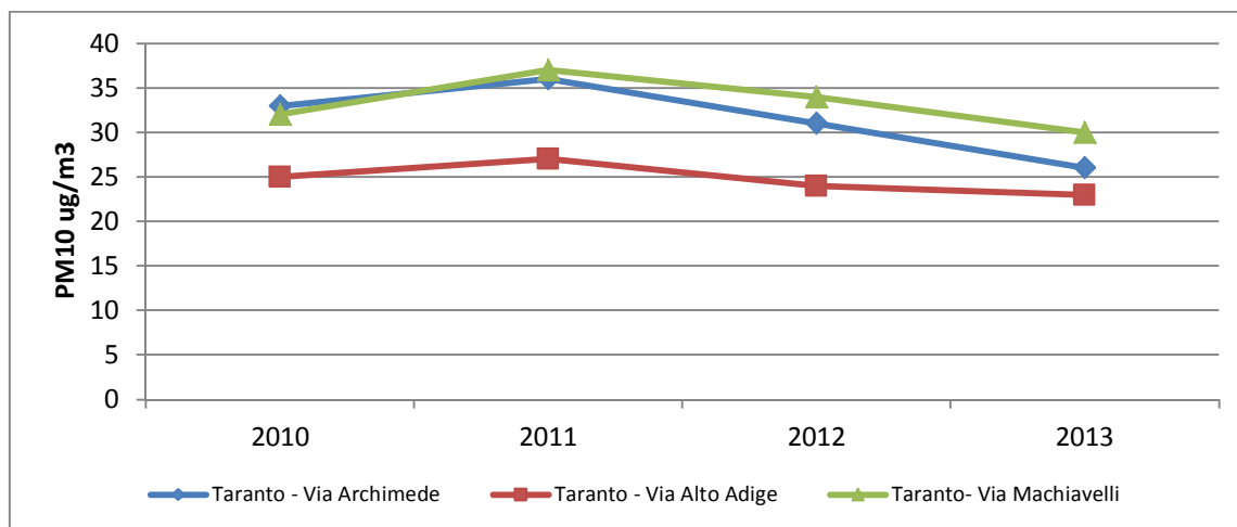
Fig.1 - Trend delle concentrazioni di PM10 dal 2010 al 2013
