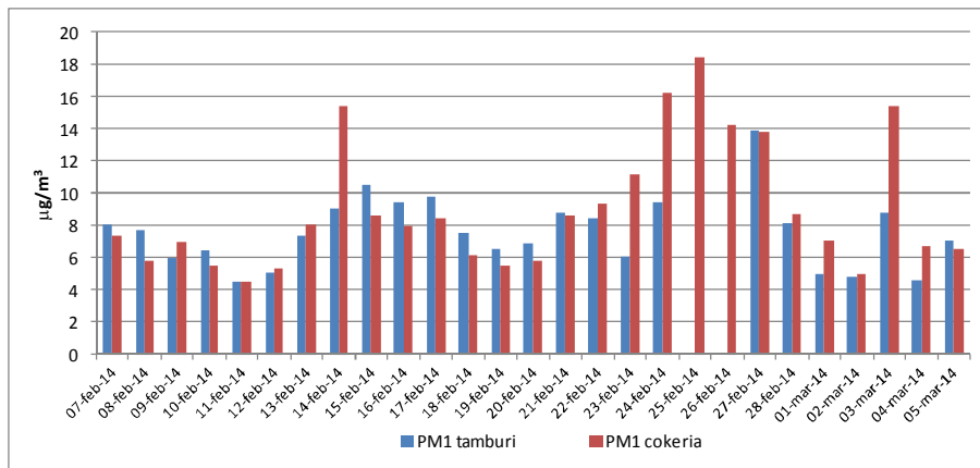
Fig.20 – Misure di PM1 Tamburi vs Cokeria
