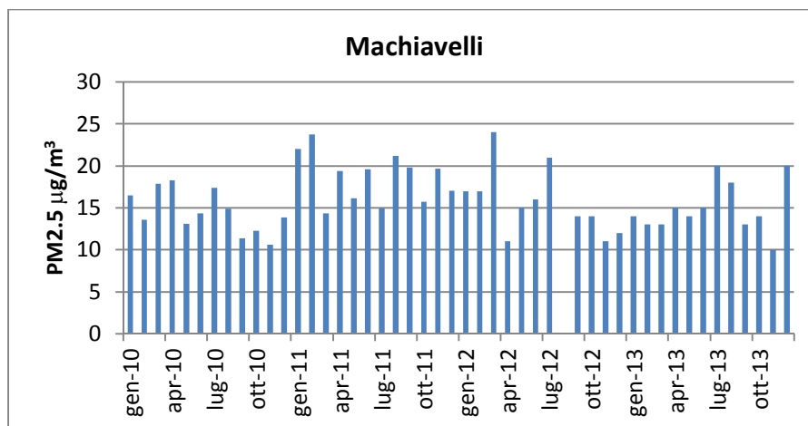
Fig.4 Medie mensili di PM2.5 - Machiavelli
