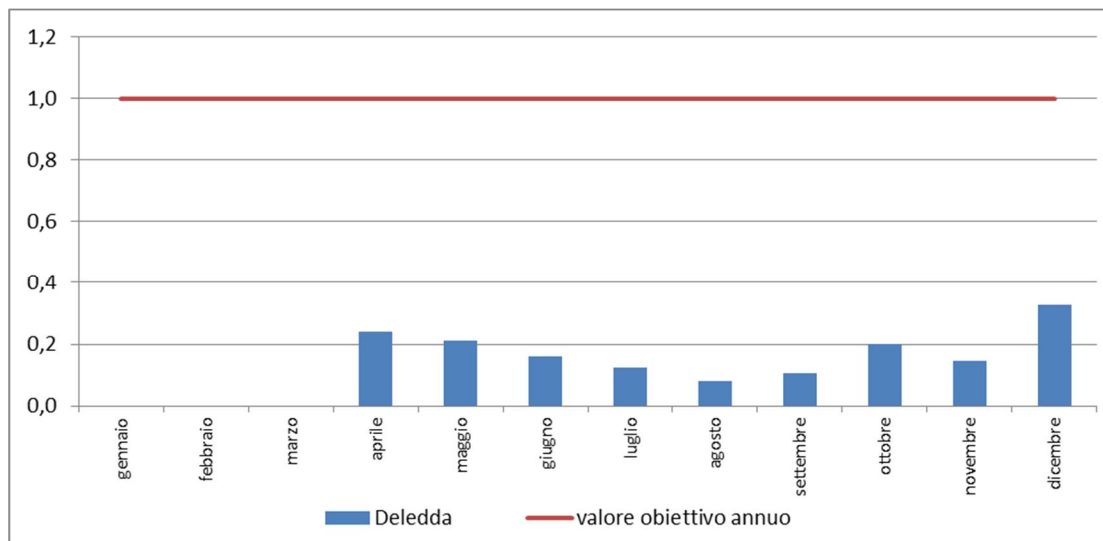
Fig.8 - Medie mensili BaP (ng/m3) Deledda anno 2013
