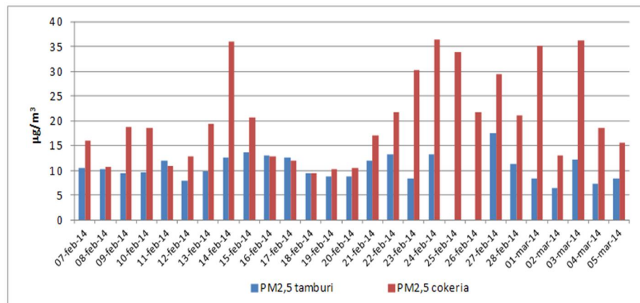
Fig.19 – Misure di PM2.5 Tamburi vs Cokeria
