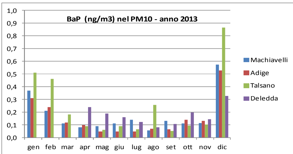
Fig.9 - Medie mensili BaP (ng/m3) Taranto anno 2013
