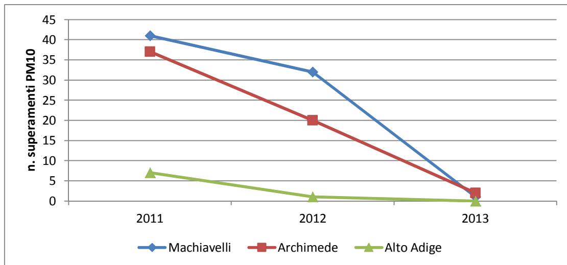
Fig.3 - Numero di superamenti di PM10 dal 2011 al 2013
