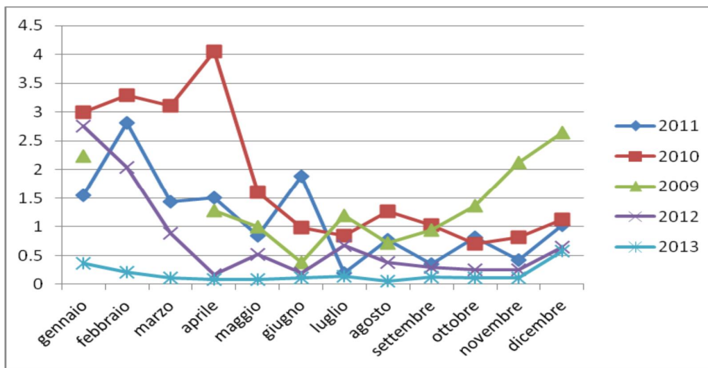
Fig.10 - Medie mensili BaP (ng/m3) in Via Machiavelli
