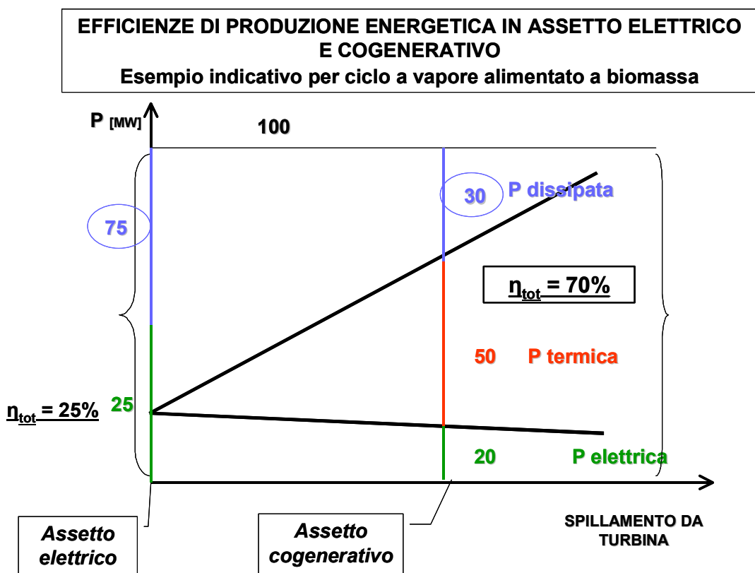
FIGURA 3: rendimento elettrico e termico di turbina a vapore da 10 MW circa.
